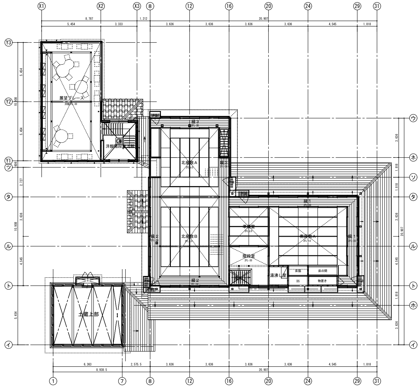
2階_平面図
