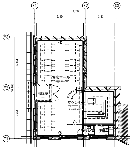
地階_平面図
