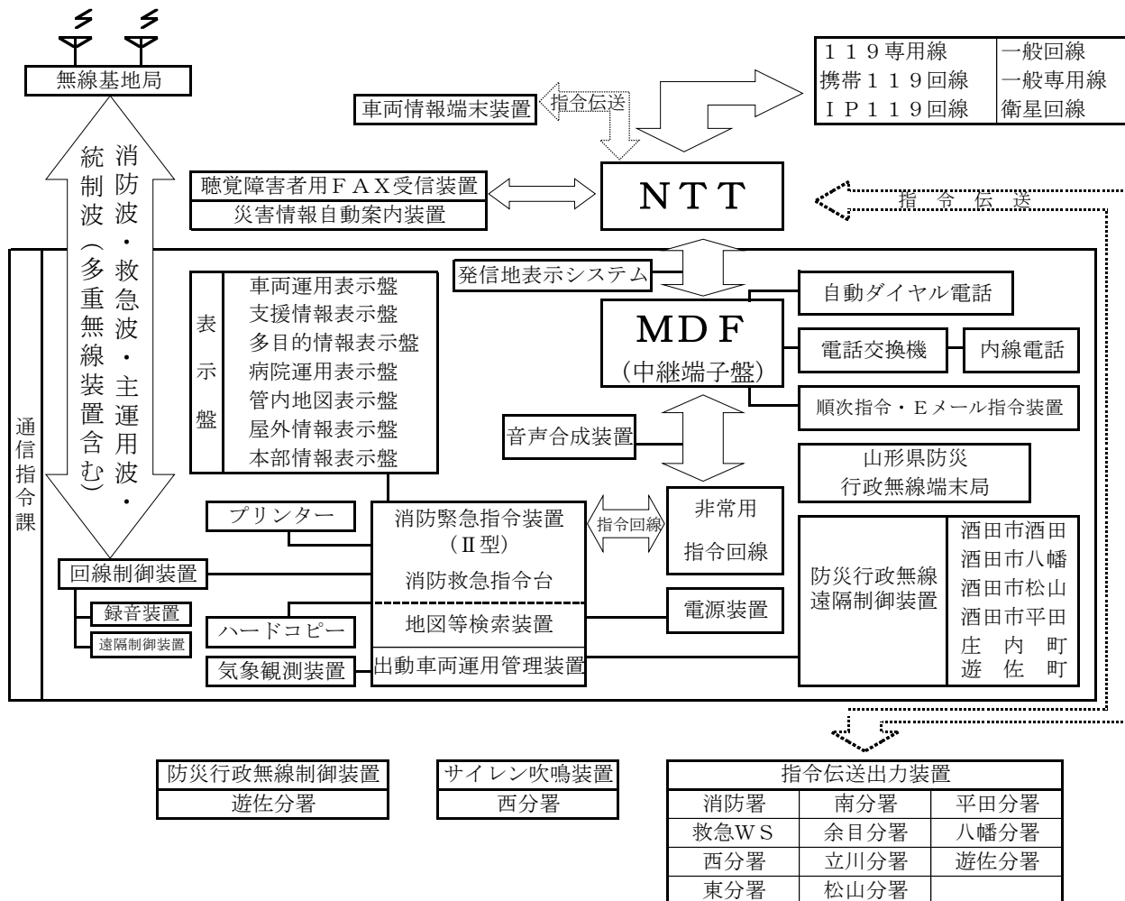
① 消防緊急通信指令系統図
