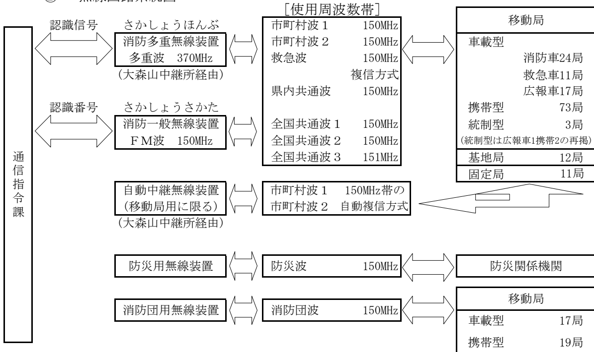
② 無線回路系統図
