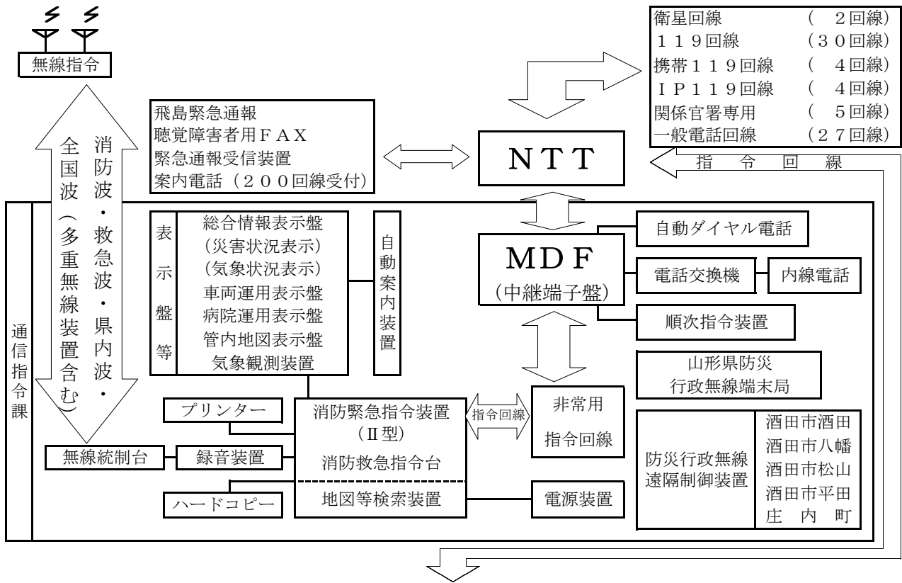
① 消防緊急通信指令系統図
