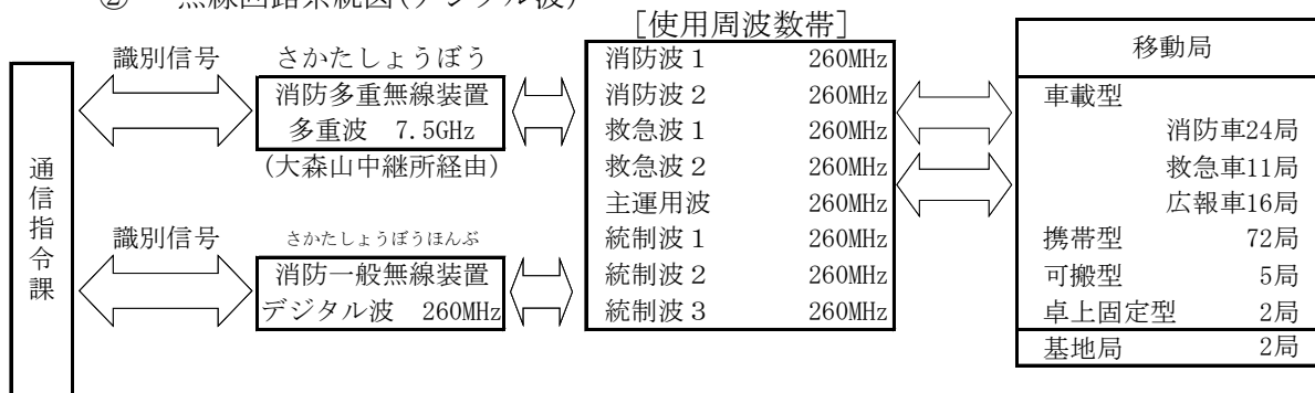
② 無線回路系統図(デジタル波)
