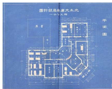
光丘文庫新築設計図（平面図）
