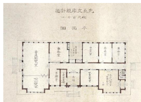
光丘文庫設計図（平面図）
