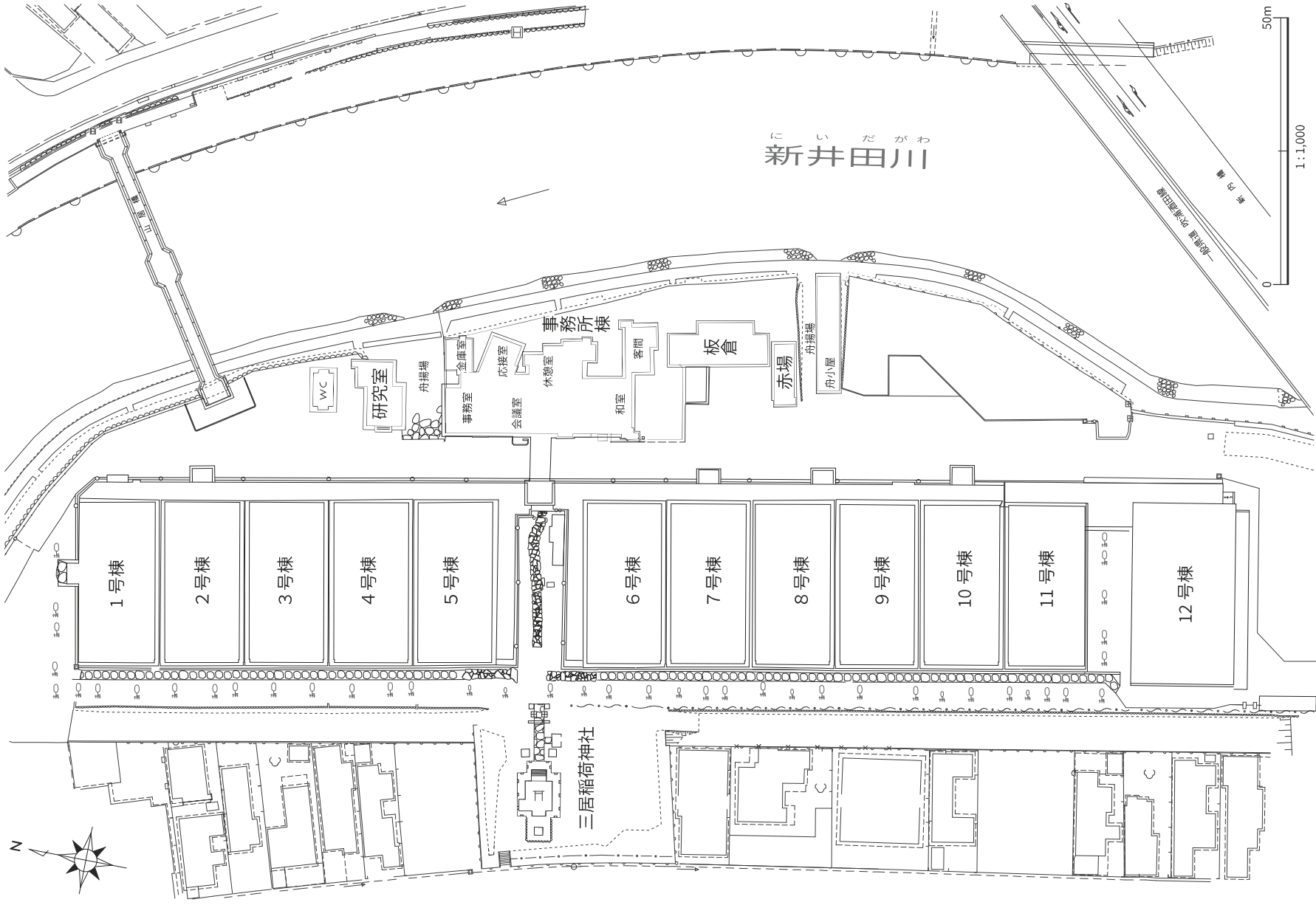
建物図面 1 全体平面図
