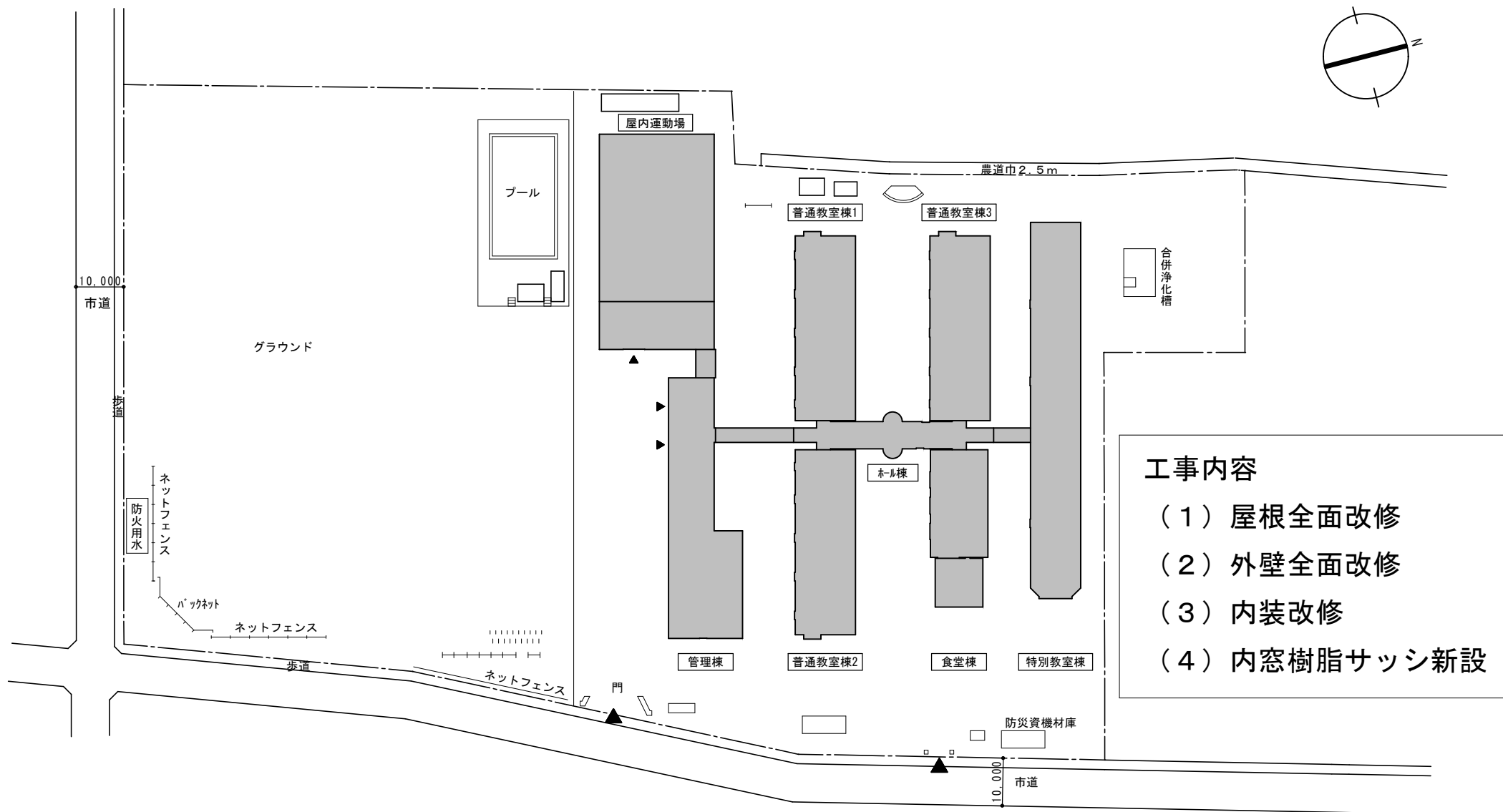
配置図
