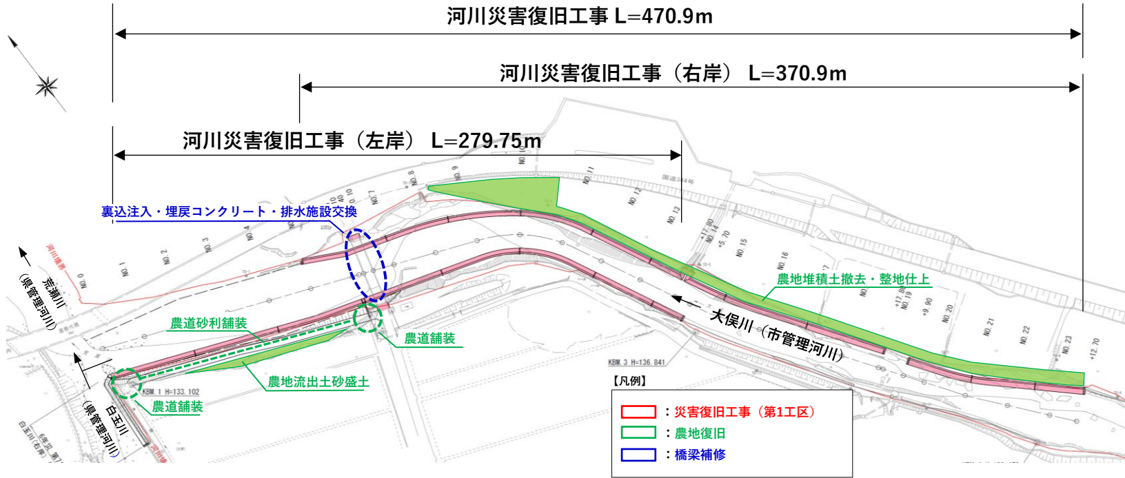
平面図
