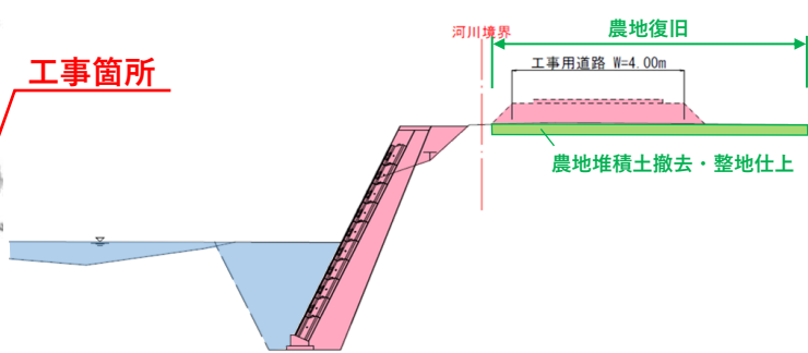
標準断面図
