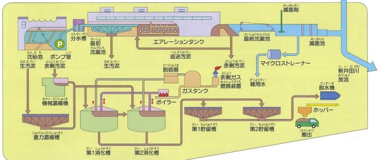
〈合流式〉
