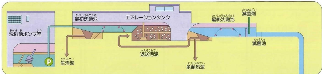
〈合流式〉
