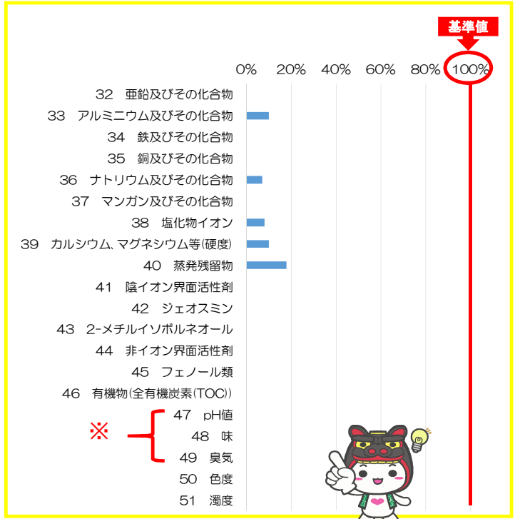
飛鳥 給水栓の水質検査結果 概要版② (グラフは直近の分析結果を基に作成しています。)
